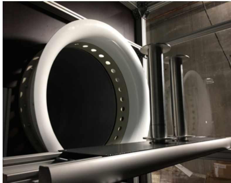
Untersuchung der Interaktion von Flettnerrotoren im Windkanal des Maritimen Technikums der Hochschule Emden/Leer
